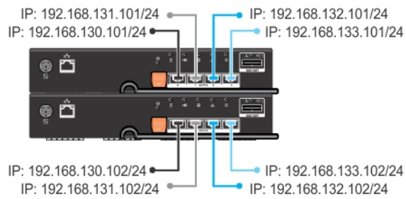
图 3: 四个群集节点连接至两台控制器
