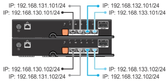
图 4: 64 台服务器连接到单个控制器
