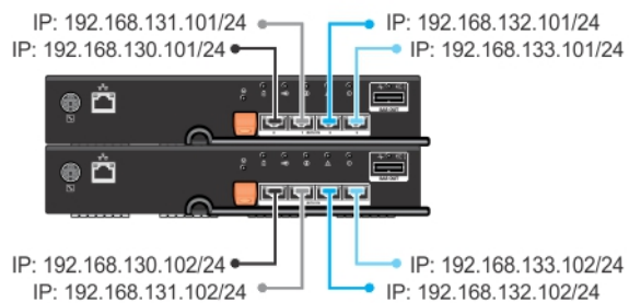
图 2: 四台主机连接到两个控制器
